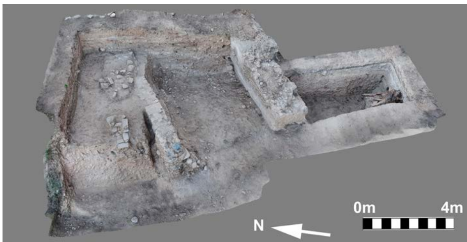
Fig. 4. Fotogrametría del estado del sondeo 3000 a fecha de mayo de 2019, vista desde el oeste. Realizada por Teresa Koffler Urbano.
